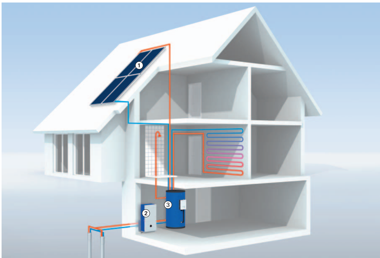
Anlagenschema Sole/Wasser-Wärmepumpe HPSol
